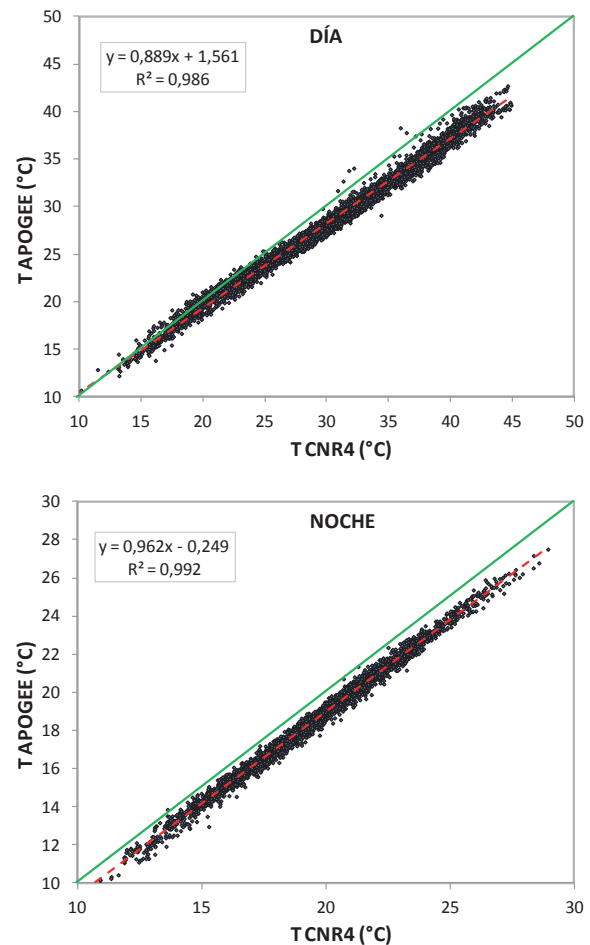
Figura 3. Comparación de las medidas realizadas con un radiómetro Apogee SI-121 y un radiómetro neto Kipp&Zonen CNR4 sobre una superficie heterogénea de viñedo, diferenciando entre día y noche.
