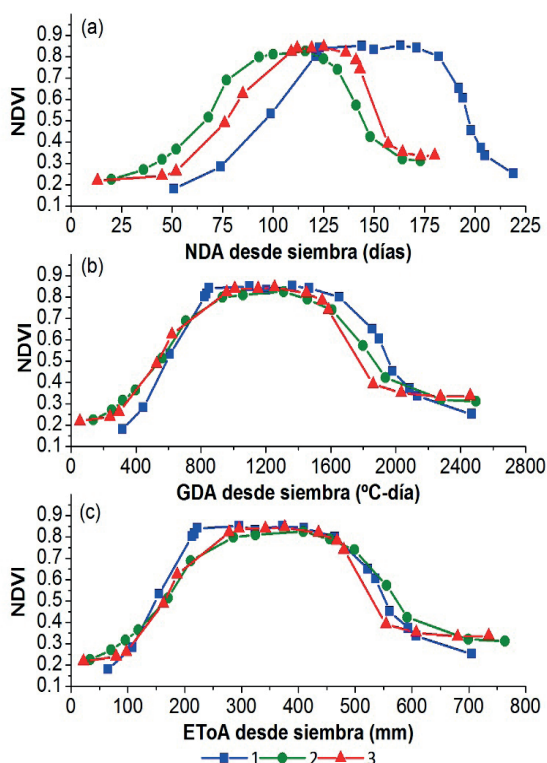
Figura 1. Curvas evolución NDVI promediado para 3 parcelas de trigo con producciones medias-altas, desde siembra a cosecha, en: (a) NDA (días); (b) GDA ( ^{\circ}C -días); (c) ET_0A (mm)
