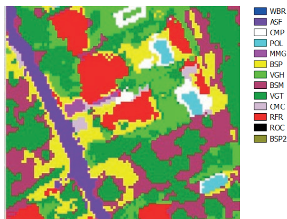
Figura 2. Detalle del resultado de la clasificación sobre una zona urbana.
