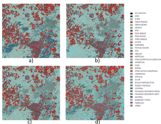
Figura 4. Aspecto visual de las clasificaciones.
