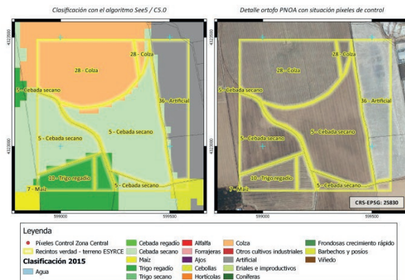
Figura 2. Aspecto visual de clasificación realizada
