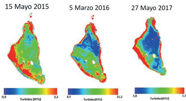
Figura 4. Mapas de turbidez (NTU).
