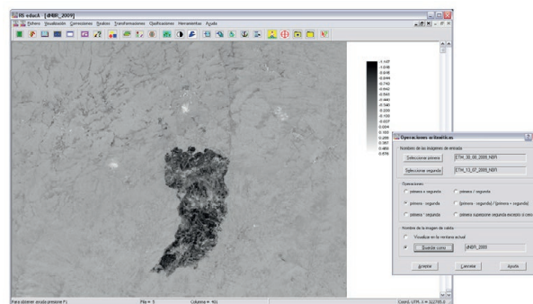
Figura 7. Imagen del Landsat dNBR.
