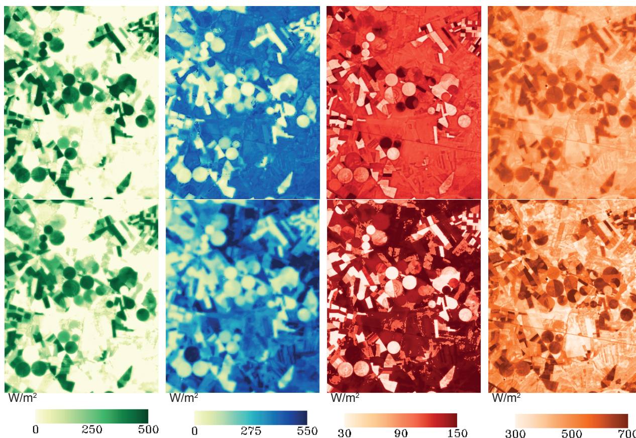
Figura 2. Resultados del balance de energía obtenido según SEBS (arriba) y METRIC (abajo). De izquierda a derecha se presenta el flujo de calor latente (LE), el flujo de calor sensible (H), el flujo de calor del suelo (G) y la radiación neta ( R_n ). Las unidades son W/m^2 .
