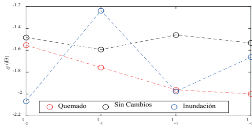
Figura 2. Tipos de variaciones temporales de \sigma_{VH} .
