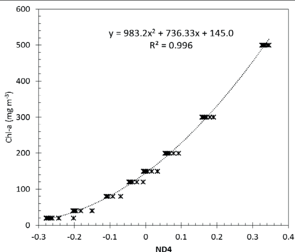
Figura 2. Calibración del modelo cuatribanda ND4.
