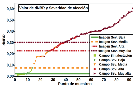
Figura 2. Gráfico que representa el valor \Delta NBR (imagen) en los puntos de muestreo, coloreados según el grado de severidad evaluado en campo. Por otro lado se marcan los umbrales ( \Delta NBR ) establecidos para clasificar la imagen en niveles de severidad.
