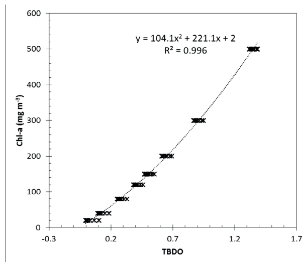
Figura 3. Calibración del modelo tribanda TBDO.
