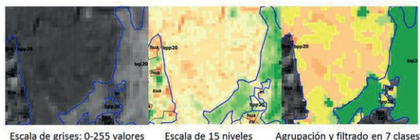
Figura 6. Ejemplo de segmentación del EVI en 7 clases.
