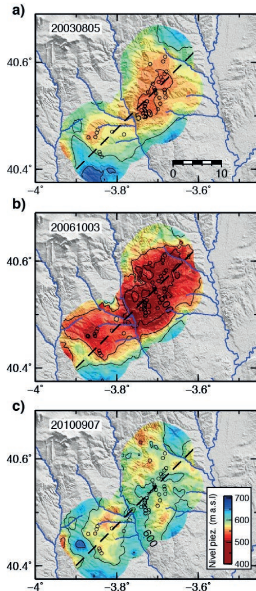
Figura 4. Mapas piezométricos para tres fechas (indicadas en cada mapa).
