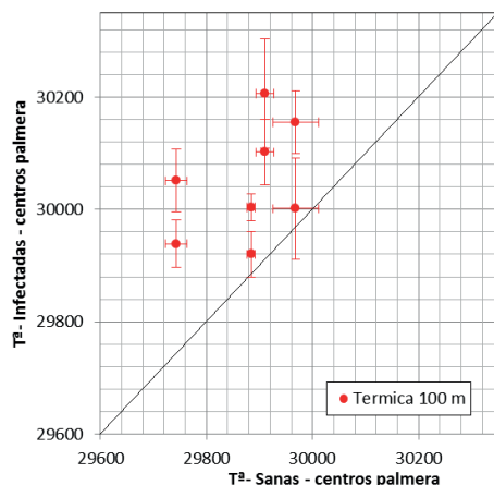
Figura 3. Comparación de los valores de Temperatura ( \times 100 ) entre palmeras sanas e infectadas por picudo.
