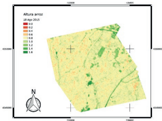
Figura 4. Mapa de las alturas de vegetación estimadas sobre la zona de estudio de Valencia el 18 de agosto de 2015. Ángulo de incidencia: 28,9°. Coordenadas UTM, Zona 30N.
