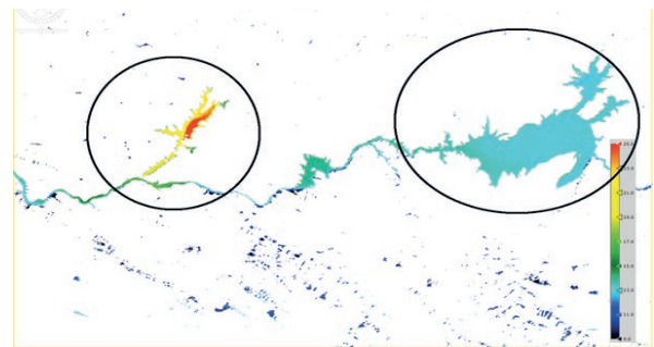
Figura 5. Vista detallada del embalse de Almaraz-Arocampo (círculo izquierdo) y el embalse de Valdecañas (círculo derecho). La leyenda permite ver la diferencia de temperatura desde el valor mínimo de 9°C hasta 25°C de la temperatura máxima.
