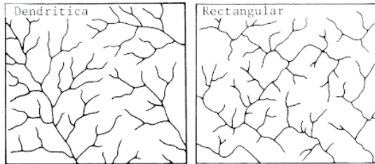
Figura 3. Disposiciones diferentes del drenaje (según Howard, 1967).
