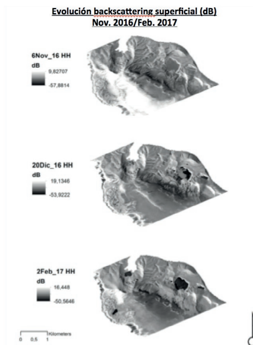
Figura 8. Muestra de la evolución del backscattering superficial del 6 de Noviembre de 2016 al 2 de Febrero de 2017, polarización HH, ángulo de incidencia 37,6°, órbita ascendente, en el área de estudio de la Isla Decepción.
