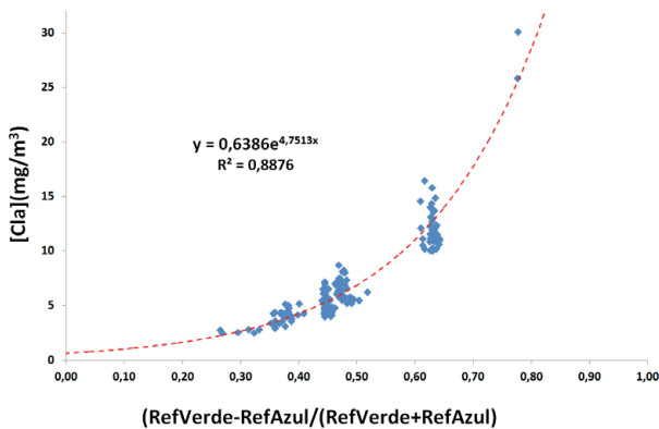
Figura 5. Relación de la los índices normalizados ( V/A ) y la clorofila- a en los puntos de muestreo del CTD.
