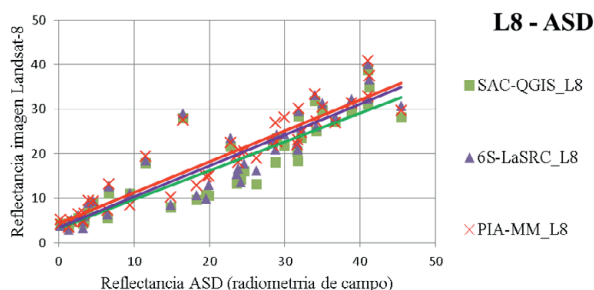
Figura 2. Correlación entre los datos de campo (eje X) y los diferentes métodos analizados: SAC-QGIS (verde), 6S-LaSRC (violeta) y PIA-MiraMon (rojo).
