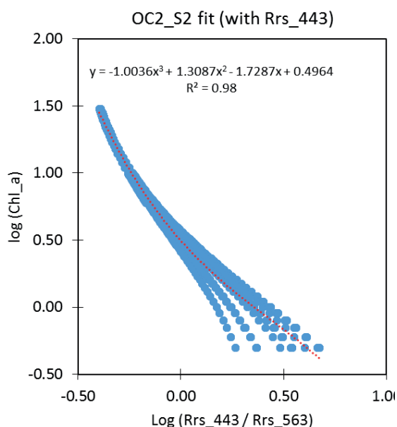
Figura 3. Calibración del algoritmo OC2 con las bandas S-2.
