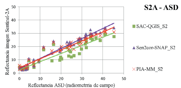
Figura 1. Correlación entre los datos de campo (eje X) y los diferentes métodos analizados: SAC-QGIS (verde), Sen2Cor-SNAP (violeta) y PIA-MiraMon (rojo).
