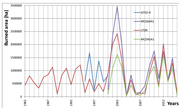
Figura 4. Distribución anual de área quemada.
