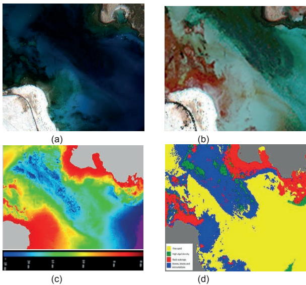
Figura 3. Resultados ARTeMISat-1 monitorización de Corralejo-Lobos: (a) Imagen corregida atmosféricamente y del reflejo solar; (b) albedo del fondo; (c) batimetría y, (d) clasificación bentónica.
