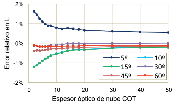
Figura 3. Errores relativos respecto a las radiancias de referencia al usar DOME con distribución-k más PCA en función del COT (eje x) y del ángulo zenital solar (leyenda).
