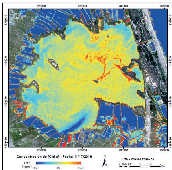
Figura 6. Mapa de concentración de [Chl-a] para el 17/11/2016.
