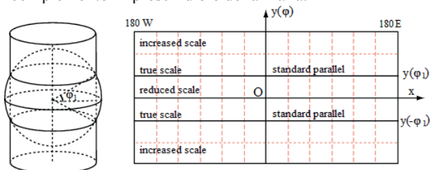
Figura 4. Proyección Mercator secante ( https://en.wikipedia.org/wiki/Mercator_projection ).
