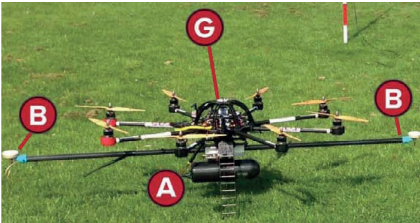
Figura 4. Componentes del sistema "TerraSystem-LidarPod"
