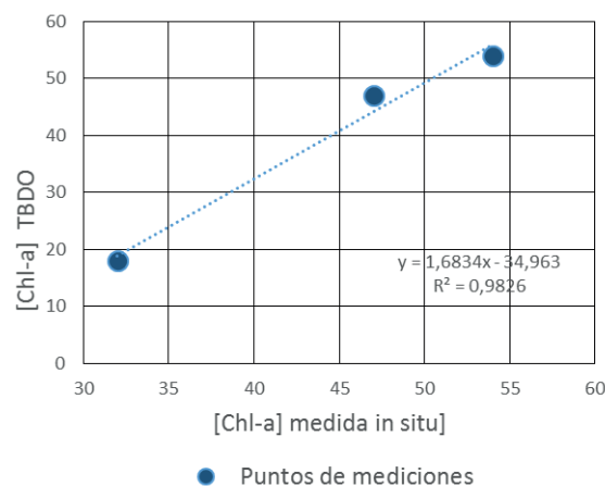
Figura 4. Relación entre [Chl-a] medida y [Chl-a] estimada por el algoritmo TBDO en el embalse de Bellús.
