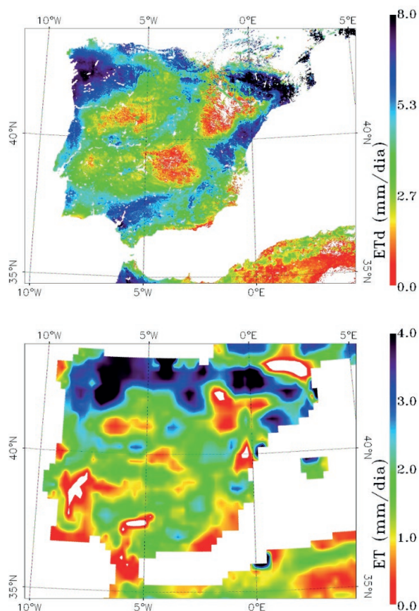
Figura 5. Mapas de evapotranspiración real diaria ( ET_d ) para la Península Ibérica estimados mediante STSEB (superior) comparado con el producto GLDAS (inferior).
