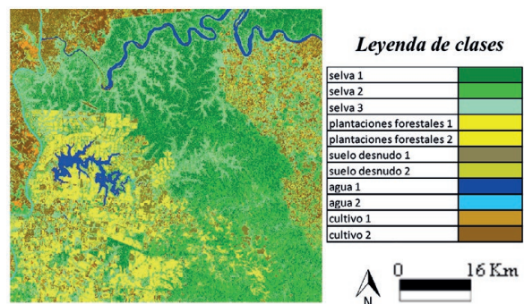
Figura 6. Clasificación supervisada imagen óptica
