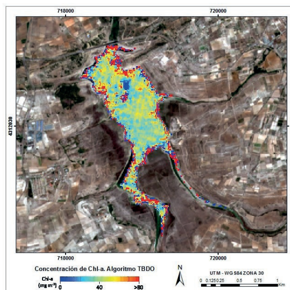
Figura 5. Mapa de clorofila aplicando el algoritmo TBDO sobre Bellús.
