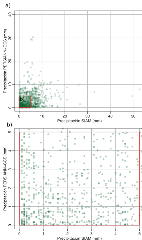
Figura 3. Gráficos de dispersión de precipitación SIAM vs. precipitación PERSIANN-CCS. a) Todos los casos en los que la precipitación de alguna fuente es mayor que 0. b) Detalle de a).
