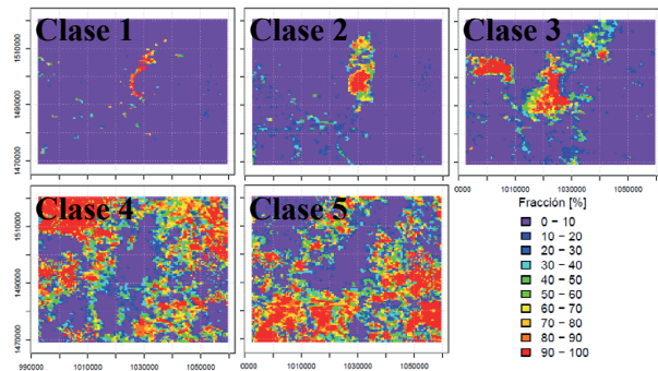
Figura 3. Fracciones de cobertura para las cinco clases puras consideradas.
