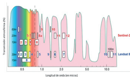
Figura 2. Comparación Sentinel 2 y Landsat 8 (modificado de Käab, 2016).
