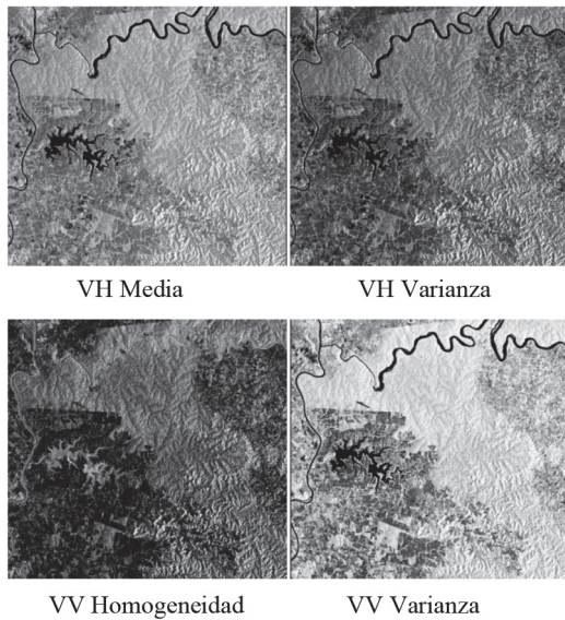
Figura 3. Bandas texturales.
