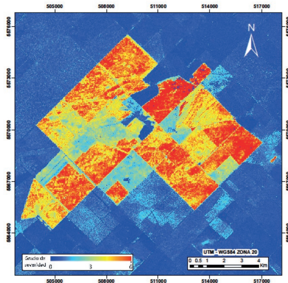
Figura 6. Mapa del grado de severidad del incendio en la zona en estudio a partir de S2.
