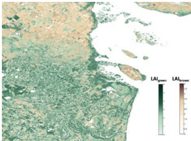
Figura 2. Mapa compuesto de LAI verde y marrón.
