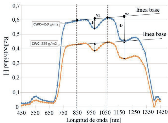
Figura 3. Representación gráfica del DWI, el cual es la suma de las profundidades a 970 y a 1200 nm, respecto a la línea base formada entre los picos a 850 y 1080 nm
