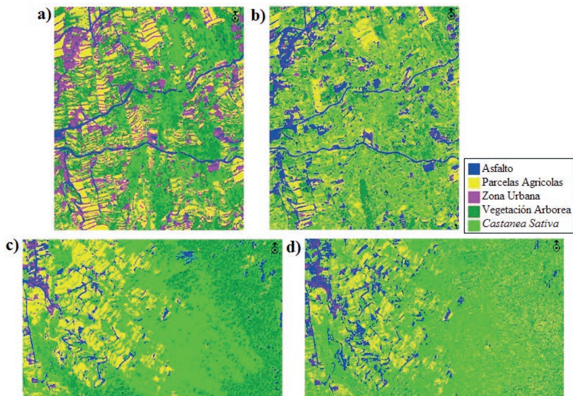
Figura 2. (a) Chasna, mes de marzo, clasificación ML. (b) Chasna multitemporal, clasificación SAM. (c) Pinolere multitemporal clasificación ANN. (d) Pinolere, mes de mayo, clasificación SAM.
