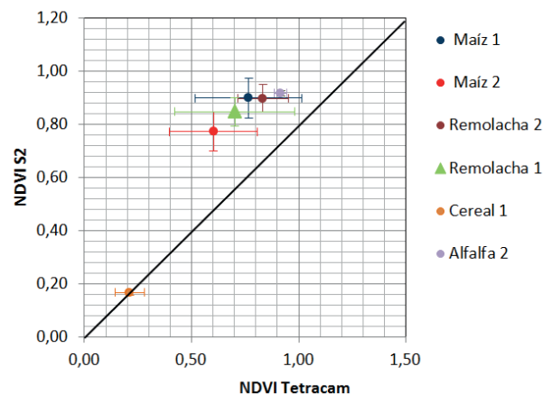
Figura 2. Comparación de los valores de NDVI derivados de Sentinel 2 y Tetracam.
