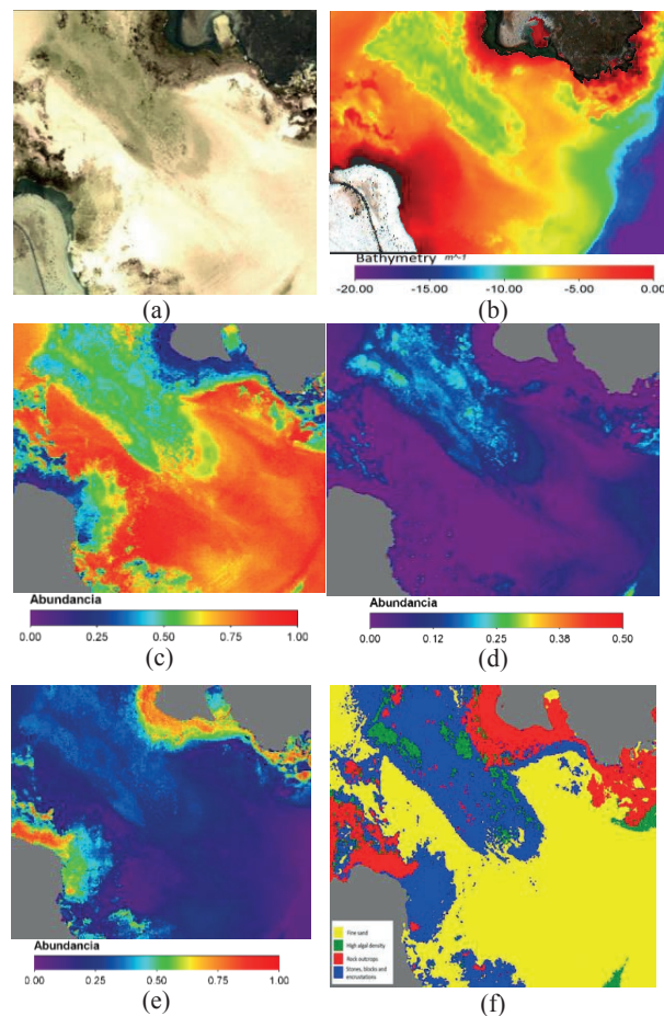
Figura 6. Resultados de la monitorización batimétrica y béntica: (a) albedo del fondo marino; (b) batimetría; (c)-(e) abundancia de arena, algas y roca sedimentaria y, (f) mapa compuesto de la cartografía bentónica.
