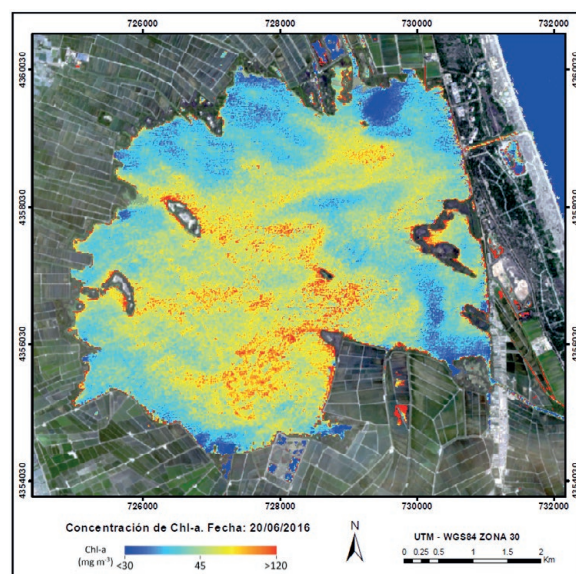
Figura 5. Mapa de concentración de [Chl-a] para el 20/06/2016.
