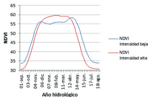
Figura 4. Curvas de NDVI de las dehesas de Q. ilex según la intensidad de sequía.
