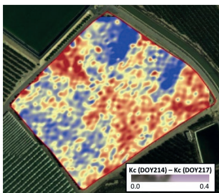
Figura 3. Mapa interpolado de la diferencia entre el K_c estimado el día 214 y 217.
