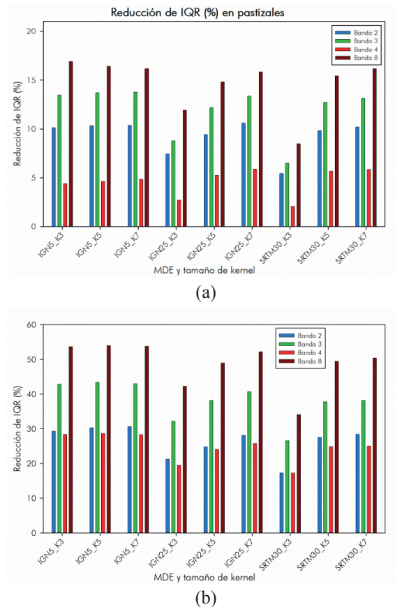
Figura 5. Reducción de IQR de dos cubiertas características, (a) Pastizales, y (b) Pino silvestre.
