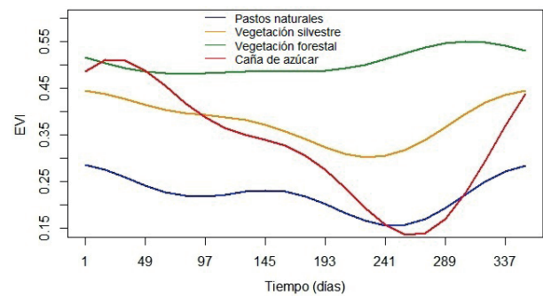
Figura 3. Curvas suavizadas de ejemplo de cuatro usos.
