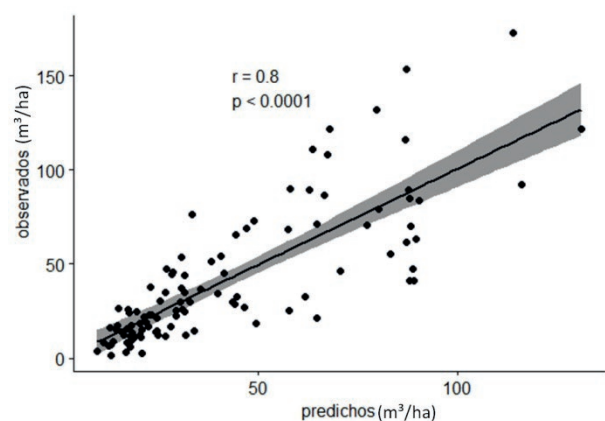
Figura 1. Observados versus predichos en la muestra de validación de volumen total para Pinus halepensis.
