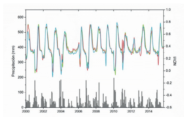
Figura 2. Perfil de NDVI y precipitación en las tres zonas estudiadas entre marzo de 2000 y septiembre de 2015. Zona 1: verde; Zona 2: rojo; Zona 3: azul.
