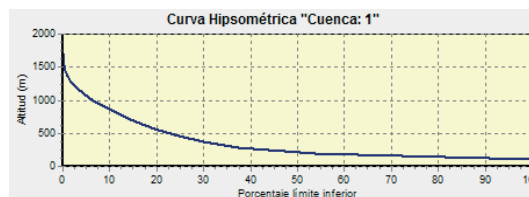
Figura 2. Curva hipsométrica.
