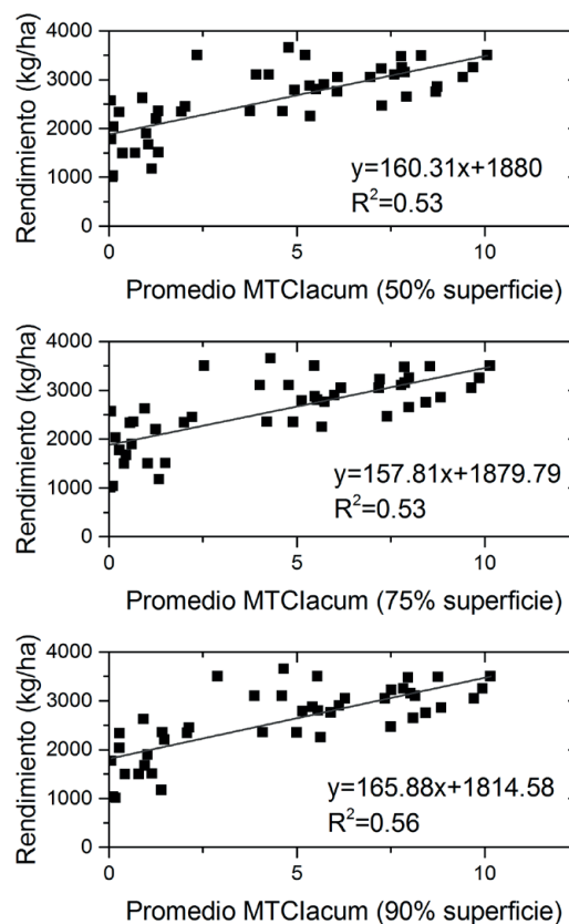
Figura 2. Diagramas de dispersión entre el rendimiento procedente del AEAP y el promedio provincial del índice MTClacum.
