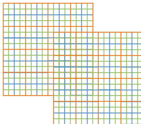
Figura 1. El alineado de los píxeles en el GSD original (los píxeles verdes de LOD= n están alineados), no asegura el alineado en los siguientes niveles de la pirámide, LOD= n-1 y LOD= n-2 (los píxeles azules y rojos están desalineados).
