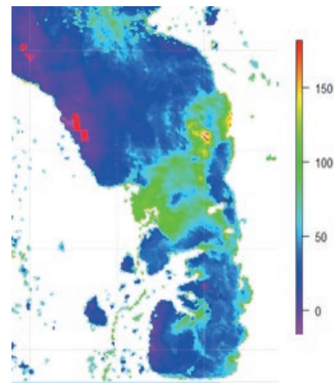
Figura 3. Aplicación del modelo a la imagen MODIS Aqua del día 28 de noviembre de 2012.
