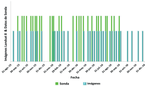
Figura 2. Serie temporal de información de las imágenes Landsat 8 y de la sonda multiparamétrica Picadas2015 en el embalse de Picadas (Septiembre 2015 – Diciembre 2016).
