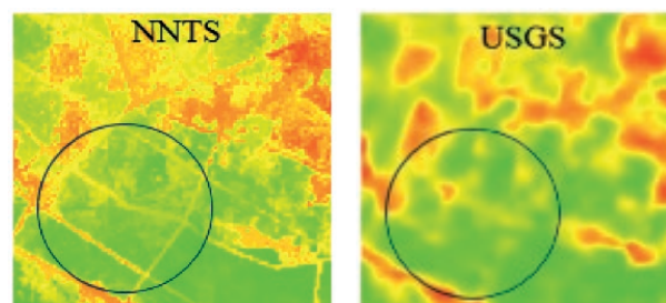
Figura 3. Imágenes TIRS de LST re-escaladas a 30 m.
