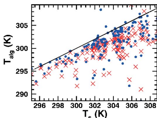
Figura 2. Valores de T_s (temperatura de la superficie) frente a T derivado a partir del algoritmo SW (puntos azules) y valores MOD11A1V6 (puntos rojos) filtrando las nubes según la QA layer . La línea 1:1 está también representada.
