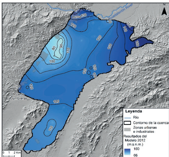
Figura 3. Estado del acuífero en 2012 según el modelo hidrogeológico desarrollado.
