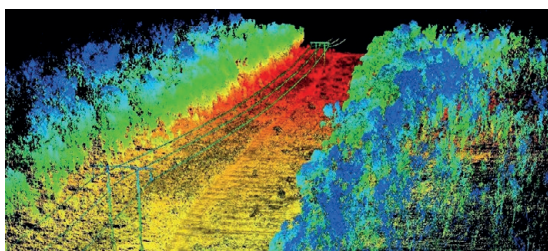
Figura 6. Red eléctrica tomada con el sistema TerraSystem-LidarPod.
