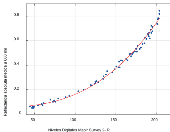
Figura 4. Curva de regresión entre valores de reflectancia y niveles digitales para el sensor R.
