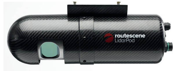
Figura 3. Sistema integrado “TerraSystem-LidarPod”
