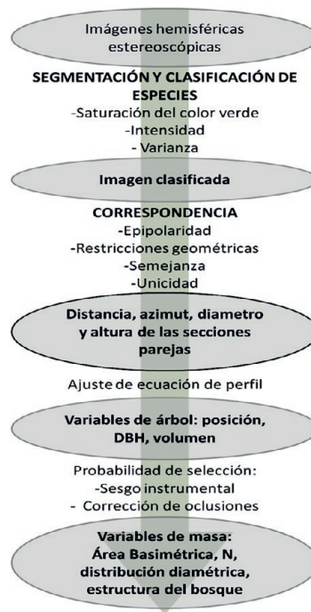
Figura 2. Esquema representando las etapas de procesamiento de imágenes obtenidas con ForeStereo.
