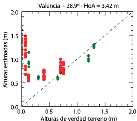
Figura 2. Comparación de las alturas estimadas con PolInSAR frente a la verdad terreno para la serie de imágenes de la zona de Valencia. Puntos rojos: arroz tipo Senia. Diamantes verdes: arroz tipo Bomba.
