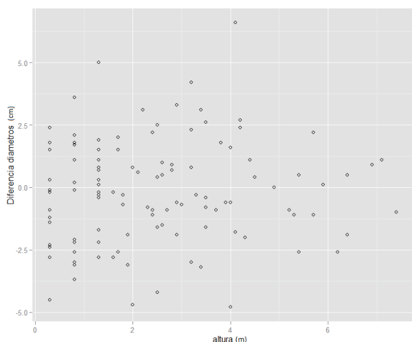
Figura 3. Relación error (cm)-altura (m).
