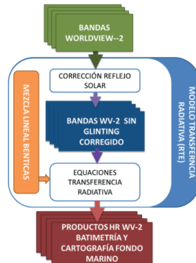
Figura 4. Diagrama procesado imágenes WorldView-2.
