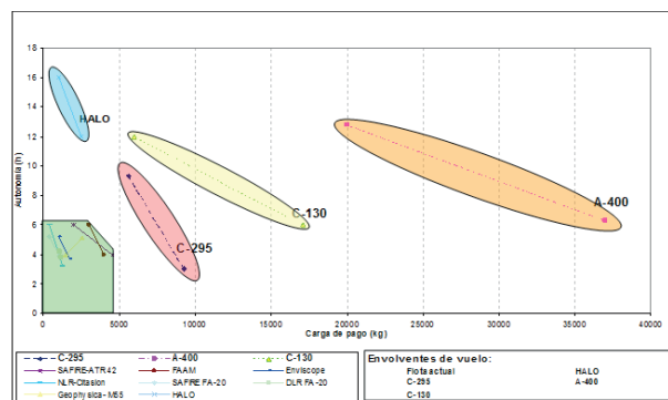
Figura 2. Autonomía vs carga útil de los aviones de la flota del consorcio EUFAR y de las tres aeronaves seleccionadas en COPAL: C-295, C-130 y A-400M.
