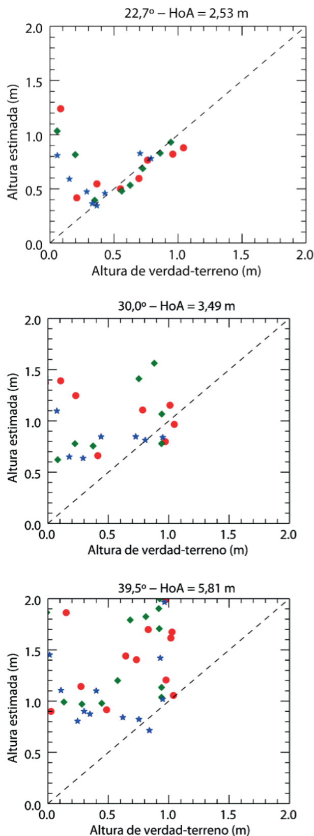
Figura 1. Comparación de las alturas estimadas con PolInSAR frente a la verdad terreno para las 3 series de imágenes de la zona de Sevilla, adquiridas con ángulos de incidencia distintos: 22,7°, 30° y 39,5°. Los símbolos corresponden a tres parcelas distintas.
